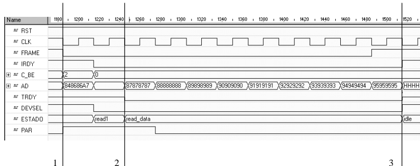
Figura 8 - Sinais do ciclo de acesso de leitura no modo burst . O sinal FRAME# permanece ativo (nível lógico 0) durante toda a fase de leitura.
